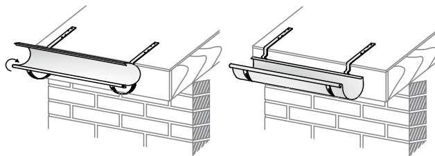
Элемент жесткости
