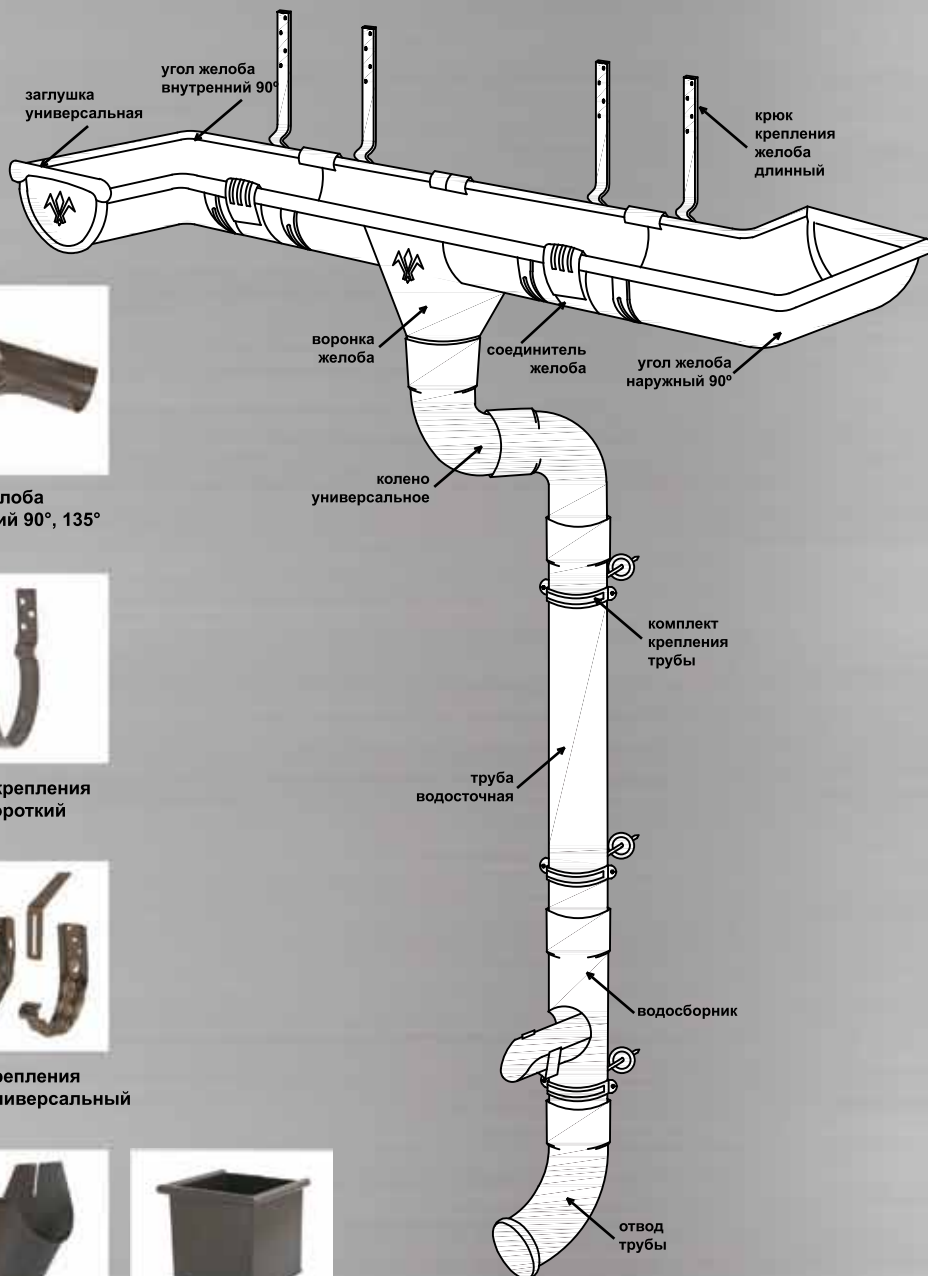
7. Заглушка универсальная 8. Заглушка полукруглая 9. Воронка желоба 10а. Воронка водосборная
