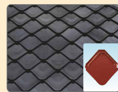
ИЗУМРУД (керамическая черепица) размер черепицы: 47,5 x 44,3 см расход на 1 кв.м: 12,5-14,0 шт.
